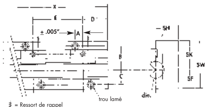
Gabarits des trous de fixation REC 62, 100 et 150 (pour galets de diamètre: 15.9, 25.4 et 38.1 mm)
