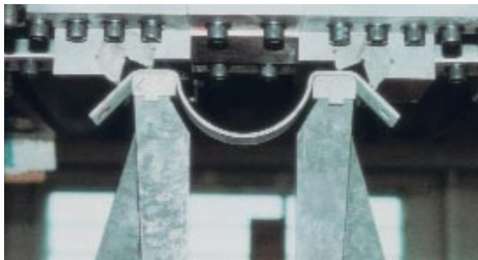
Pliage bride en acier (HLE) pour l'industrie navale.
