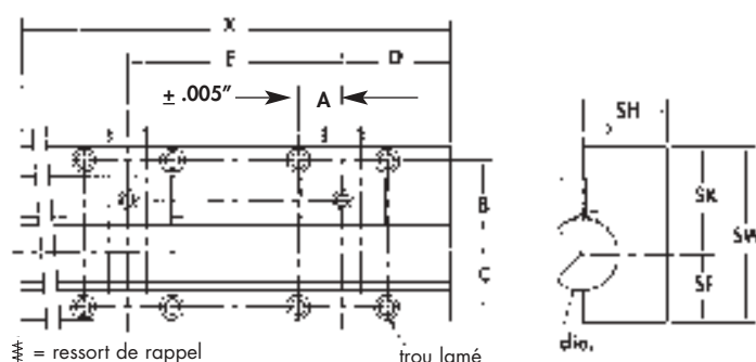
Gabarits des trous de fixation REC 200, 250 et 300 (pour galets de diamètre: 50.8, 63.5 et 76.2 mm)
